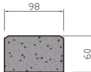
SECCIÓN TRANSVERSAL A-A
