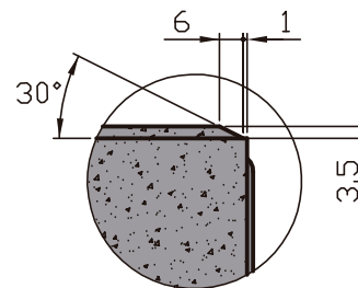
SECCIÓN TRANSVERSAL A-A
